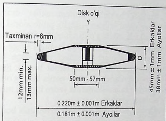
Diskning umumiy ko'rinishi va o'lchamlari.
