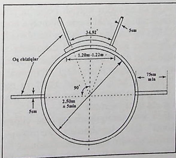
Disk uloqtirish joyi o'lchamlari.
