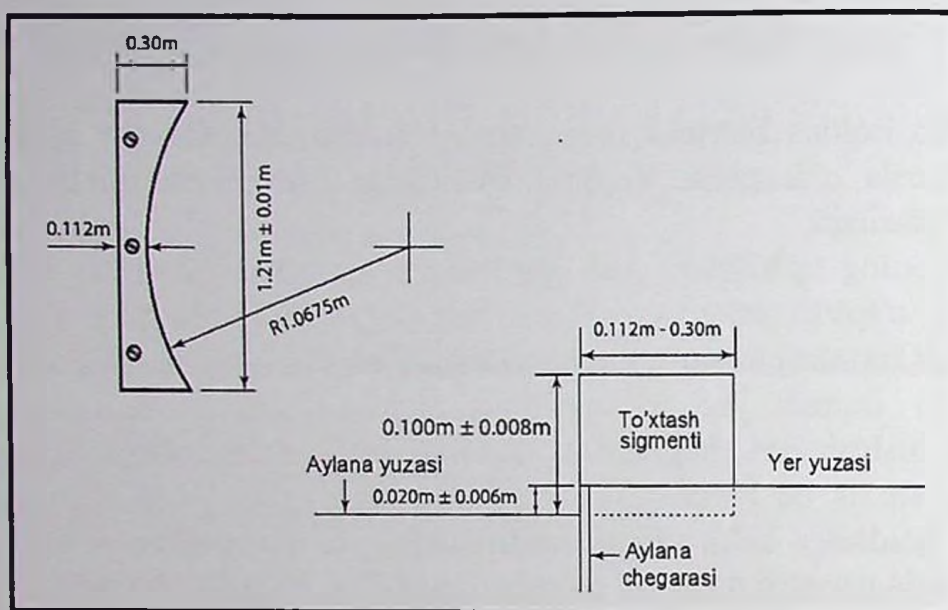
Yadro itqitish joyini o'lchamlari
