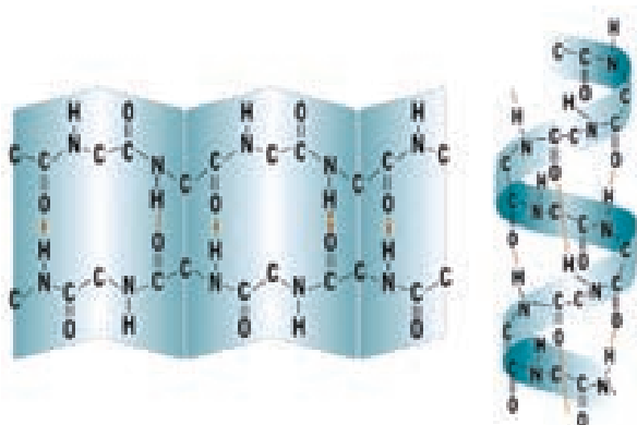
Ikkilamchi struktura
