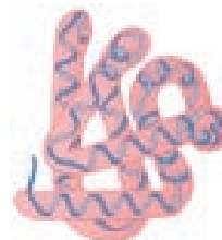
Uchlamchi struktura
