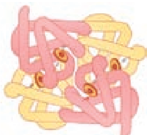
To'rtlamchi struktura
