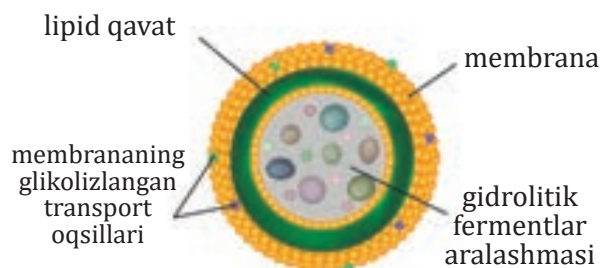
2.16-rasm. Lizosoma
