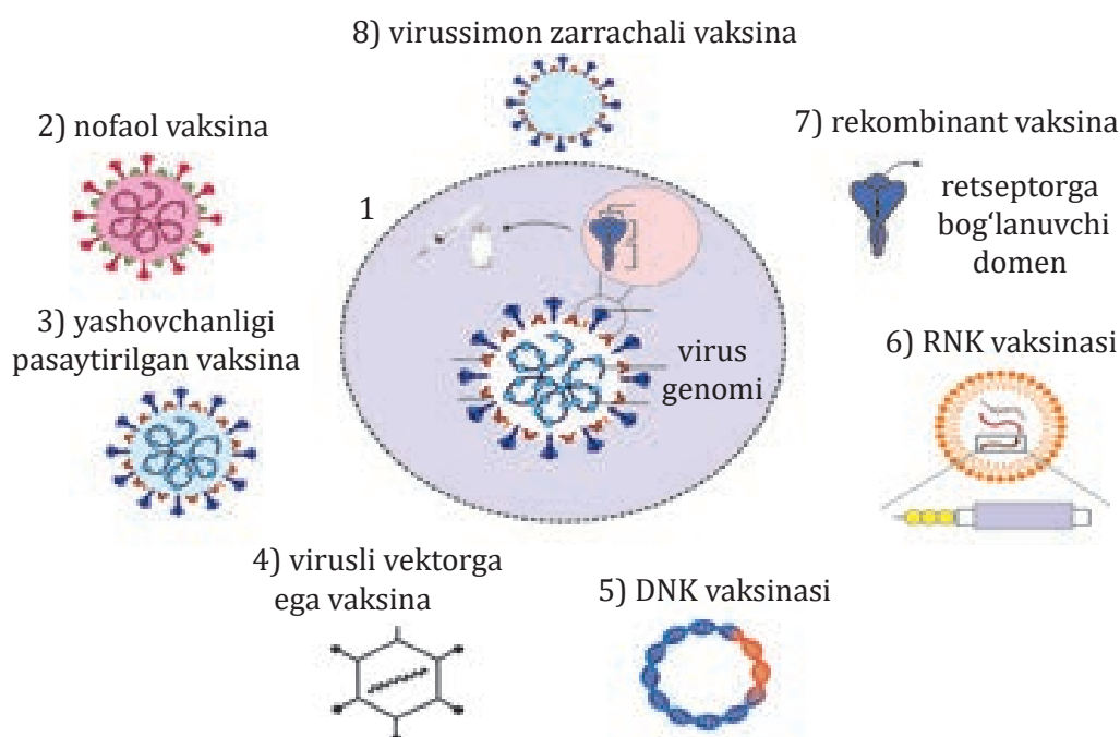
5.9-rasm. Vaksinalar
